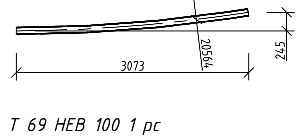
T 69 HEB 100 1 pc M 1:50
