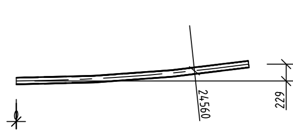
T 71 HEB 100 1 pc M 1:50
