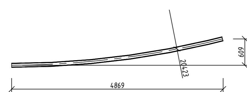
T 140 HEB 100 1 ks M 1:50
