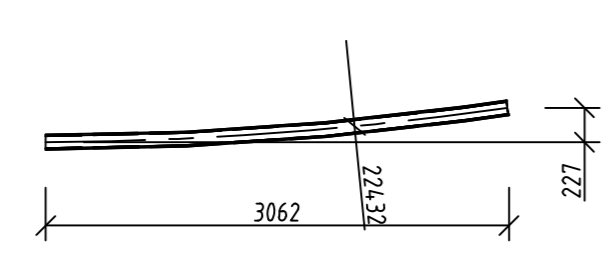
T 64 HEB 100 1 ks M 1:50
