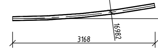
T 74 HEB 100 1 pc M 1:50
