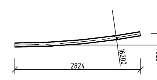
T 55 HEB 100 1 pc M 1:50
