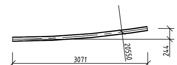
T 66 HEB 100 1 ks M 1:50
