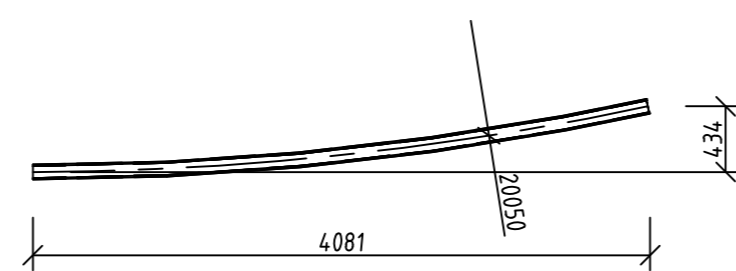
T 109 HEB 100 1 pc M 1:50
