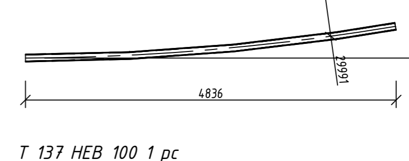
T 137 HEB 100 1 pc M 1:50
