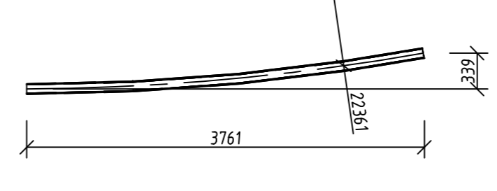
T 115 HEB 100 1 pc M 1:50
