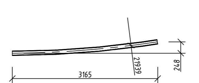
T 73 HEB 100 1 ks M 1:50
