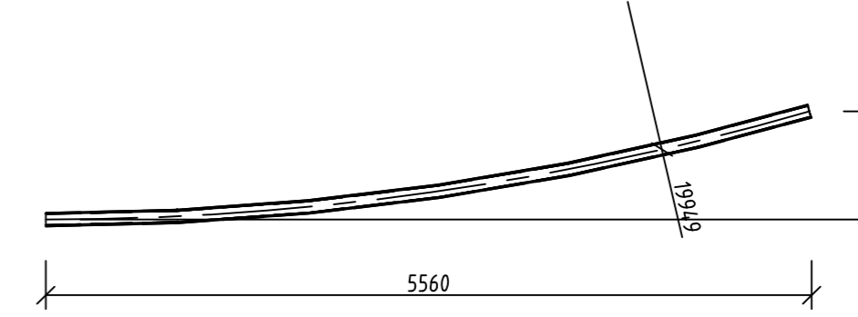
T 144 HEB 100 1 pc M 1:50
