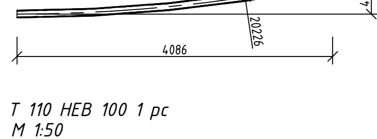
T 110 HEB 100 1 pc M 1:50
