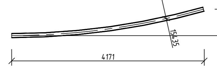
T 127 HEB 100 1 pc M 1:50
