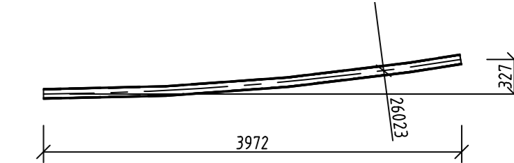
T 102 HEB 100 1 pc M 1:50
